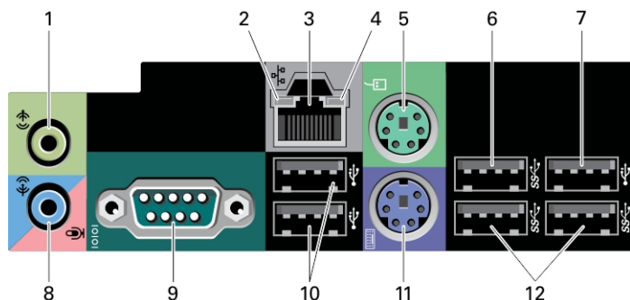
Obrázek 2. Pohled na zadní panel pracovní stanice T3610/T5610
